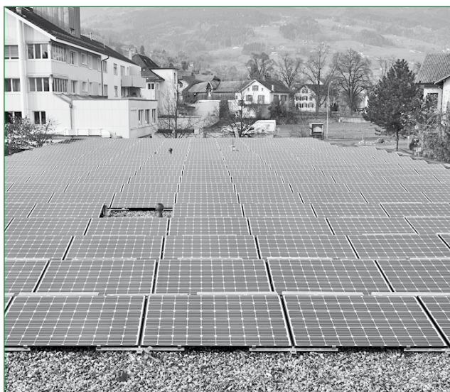
Fertig erstellte PV-Anlage auf dem EW-Gebäude
